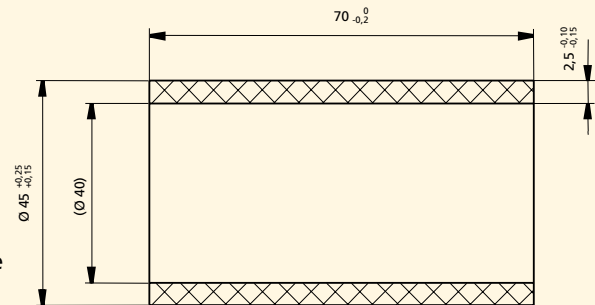
Bild 1: Beispiel für die Tolerierung einer Lagerbuchse
